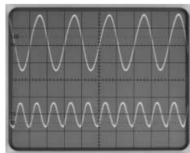
Foto: 50MHz und 100MHz Sinus-Signal mit alternierender Triggrung
